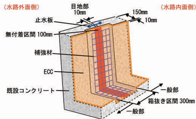
(a) 概略図
