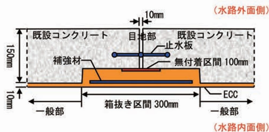
(b) 断面図
