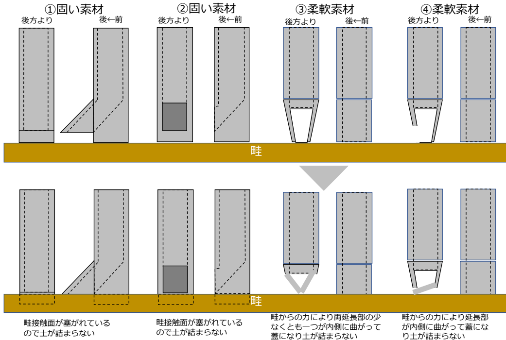
図2 新技術の播種ノズルの背面図（左）と側面図（右）、畦に接触した状態（上）と強く当たった状態（下）
