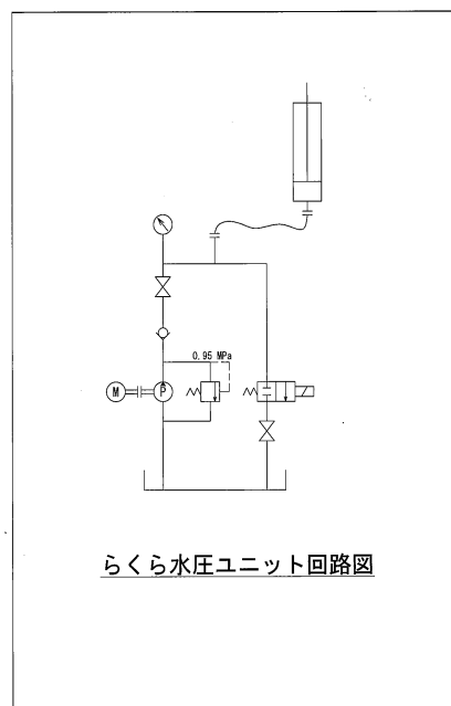
基本構成例（水圧回路のみ）
