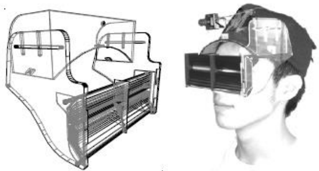
図 中心視野を制限するために用いる実験装置の構造
